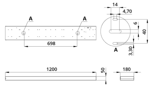
Монтаж светильника
