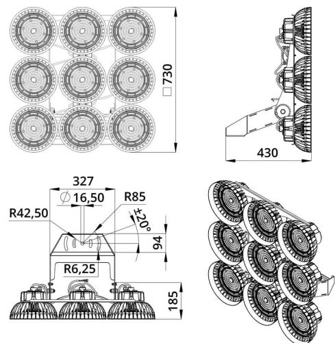
Габаритный чертёж
