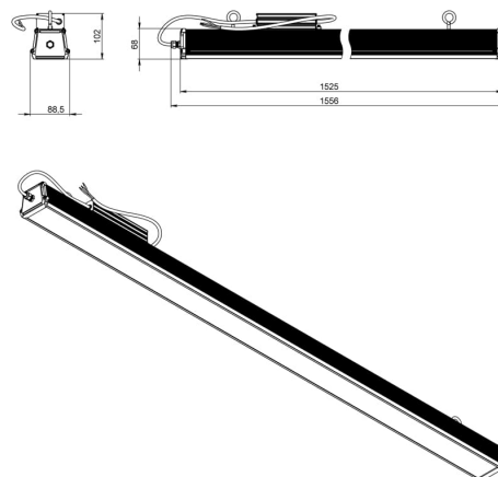
Габаритный чертеж
