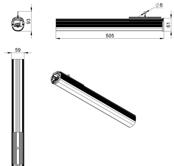
Габаритный чертеж
