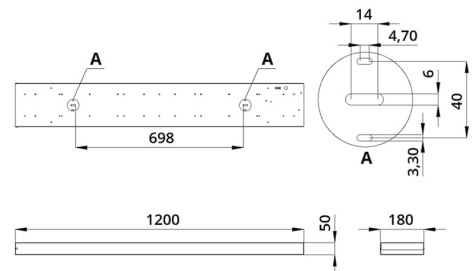
Монтаж светильника
