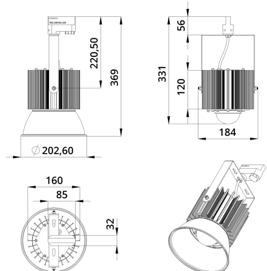
Габаритный чертёж
