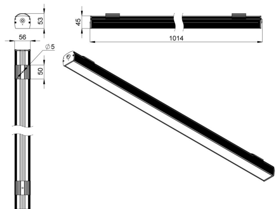
Габаритный чертеж
